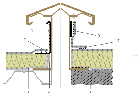
Рис. 7.13. Примыкание пароизolyatsionnogo ROCKbarrier и гидроизolyatsionnogo ROCKmembrane к выступающим элементам на покрытии.
