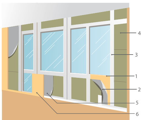
Рис. 1.5. Каркасная стена:
