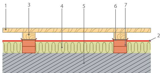
Рис. 4.5. Утепление плитного перекрытия с лагами по столбикам: 1 — покрытие пола; 2 — пароизоляция ROCKWOOL; 3 — лага; 4 — плиты ROCKWOOL ЛАЙТ БАТТС® или Лайт Баттс СКАНДИК требуемой толщины; 5 — плита перекрытия; 6 — прокладка из рубероида; 7 — столбик из кирпича или бруска из легкого бетона.
