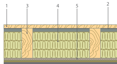
Рис. 4.2. Утепление перекрытия по деревянным балкам над холодным подвалом: 1 — покрытие пола из досок или паркетных щитов; 2 — пароизоляция ROCKWOOL; 3 — деревянные балки, опирающиеся на цоколь или стены подвала; 4 — плиты ROCKWOOL ЛАЙТ БАТТС® или Лайт Баттс СКАНДИК требуемой толщины; 5 — обшивка из досок или листовых материалов.
