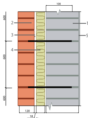
Рис. 1.16. Трехслойная кирпичная стена с утеплением плитами ROCKWOOL КАВИТИ БАТТС®: 1 — внутренняя часть стены; 2 — наружная защитно-декоративная кладка толщиной 120 мм; 3 — воздушный зазор; 4 — плиты ROCKWOOL КАВИТИ БАТТС®; 5 — внутренняя штукатурка.
