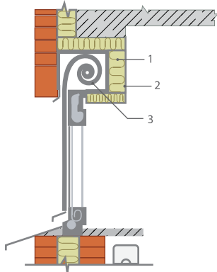
Рис. 1.14. Утепление полости для свернутых роль-ставней: 1 — плиты ROCKWOOL ЛАЙТ БАТТС® или Лайт Баттс СКАНДИК; 2 — внутренняя отделка утепляющего короба; 3 — роль-ставни.
