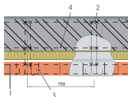
Рис. 1.17. Соединение несущей части трехслойной стены с декоративно-защитной кирпичной кладкой арматурной сеткой и гибкими связями: 1 — арматурная сетка; 2 — гибкие связи в форме петли; 3 — вязальная проволока; 4 — арматурный стержень.
