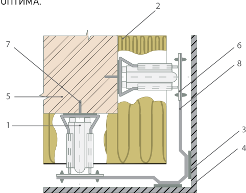
Рис. 1.27. Схема крепления облицовки и плит ROCKWOOL ВЕНТИ БАТТС® в зоне наружного угла здания: 1 — кронштейн; 2 — плиты ROCKWOOL ВЕНТИ БАТТС® или ROCKWOOL ВЕНТИ БАТТС Д®; 3 — кляммер; 4 — плитка облицовочная; 5 — утепляемая стена; 6 — заклепка; 7 — анкерный дюбель; 8 — гнутый уголкового профиль.
