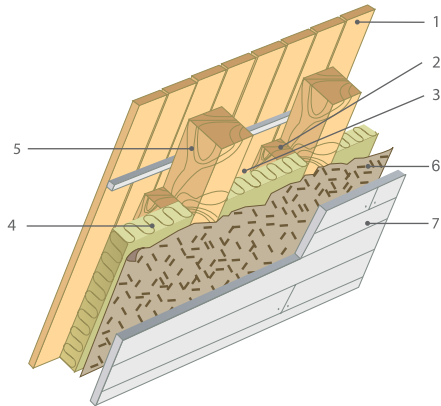
Рис. 7.2. Покрытие мансарды:
