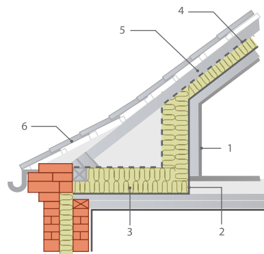
Рис. 7.6. Установка изоляционного материала по всей поверхности конструкций, граничащих с наружной средой: 1 — внутренняя обшивка; 2 — пароизоляция ROCKWOOL; 3 — плиты ROCKWOOL ЛАЙТ БАТТС® или Лайт Баттс СКАНДИК; 4 — мембрана ROCKWOOL для кровель; 5 — стропильная нога; 6 — покрытие кровли.
