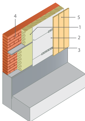
Рис. 1.8. Устройство вентилируемой воздушной прослойки в стенах с обшивкой сайдингом: 1 — плиты ROCKWOOL ЛАЙТ БАТТС® или Лайт Баттс СКАНДИК®; 2 — мембрана ROCKWOOL для стен; 3 — вентилируемая воздушная прослойка; 4 — внутренняя стенка; 5 — наружная обшивка.
