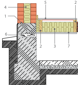
Рис. 4.1. Устройство продухов для вентиляции подполья: 1 — гидроизоляция; 2 — несущая балка перекрытия; 3 — плиты ROCKWOOL ЛАЙТ БАТТС® или Лайт Баттс СКАНДИК; 4 — плиты ROCKWOOL КАВИТИ БАТТС®; 5 — пол; 6 — вентиляционный продух; 7 — подшивка потолка подвала.
