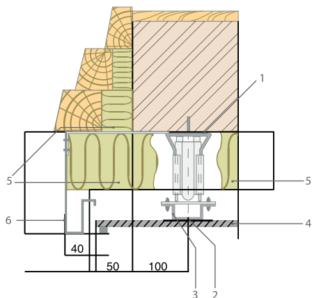
Рис. 1.26. Узел примыкания навесной фасадной системы к оконному проему: 1 — кронштейн; 2 — направляющая; 3 — кляммер; 4 — плитка облицовочная; 5 — плита ROCKWOOL ВЕНТИ БАТТС® или ВЕНТИ БАТТС Д®; 6 — стальной элемент рамы оконного обрамления толщиной 0,55 мм.
