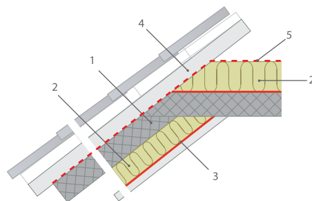
Рис. 7.7. Дополнительное утепление мансарды: 1 — существующая теплоизоляция; 2 — дополнительный слой утеплителя ROCKWOOL ЛАЙТ БАТТС® или Лайт Баттс СКАНДИК; 3 — пароизоляция ROCKWOOL; 4 — вентилируемая воздушная прослойка; 5 — мембрана ROCKWOOL для кровель
