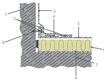
Рис. 7.17. Примыкание системы ROCKROOF к вертикальной стене и водосточной воронке 1 — парапет; 2 — герметик; 3 — ПВХ мембрана ROCKmembrane; 4 — ламинированная ПВХ жесь; 5 — ПВХ мембрана ROCKmembrane; 6 — плиты ROCKWOOL РУФ БАТТС ЭКСТРА®, РУФ БАТТС ОПТИМА®, РУФ БАТТС В+Н®; 7 — основание кровли; 8 — пароизоляция ROCKbarrier; 9 — механическое крепление ПВХ жести
