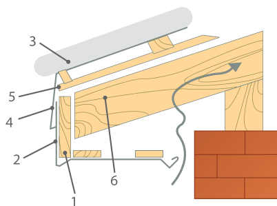
Рис. 7.5. Устройство продухов в подшивке карниза: 1 — карнизная доска; 2 — карнизная подшивочная планка; 3 — кровельное покрытие; 4 — карнизная планка; 5 — контробрешетка; 6 — стропильная нога.
