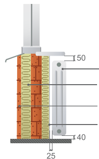
Рис. 1.15. Установка отопительного прибора: 1 — отопительный прибор; 2 — плиты ROCKWOOL ЛАЙТ БАТТС® или Лайт Баттс СКАНДИК; 3 — наружная стена; 4 — глянцевая алюминиевая фольга.
