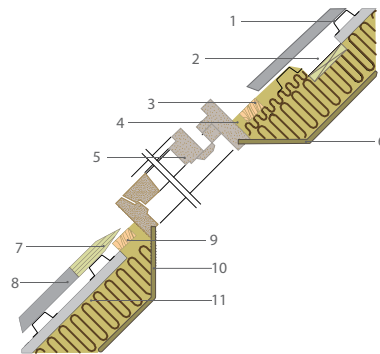
Рис. 7.8. Установка оконных блоков для освещения мансардных помещений: 1 — обрешетка; 2 — дренажный желоб; 3 — монтажный брус; 4 — верхняя секция оклада; 5 — мансардное окно; 6 — внутренняя отделка проема; 7 — нижняя секция оклада; 8 — кровельное покрытие; 9 — монтажный брус; 10 — внутренняя отделка проема; 11 — плиты ROCKWOOL ЛАЙТ БАТТС® или Лайт Баттс СКАНДИК
