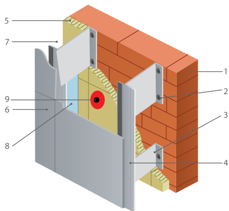
Рис. 1.25. Конструкция навесного фасада с воздушным зазором: 1 — утепляемая стена; 2 — распорный анкер; 3 — кронштейн; 4 — направляющие; 5 — плиты серии ВЕНТИ БАТТС®; 6 — плиты защитной декоративной облицовки (например, ROCKPANEL); 7 — воздушный зазор; 8 — вставка кронштейна; 9 — фасадный дюбель.
