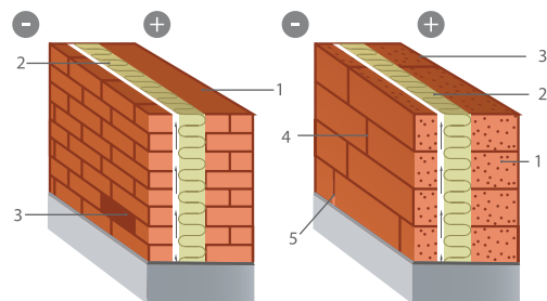
Рис. 1.9. Устройство вентиляционных продухов в кирпичной стенке: 1 — внутренняя стенка трехслойной стены; 2 — плиты ROCKWOOL КАВИТИ БАТТС®; 3 — кирпич, поставленный на ребро; 4 — шов, заполненный раствором; 5 — шов, незаполненный раствором.
