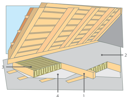
Рис 5.1. Чердачное перекрытие, утепленное плитами ROCKWOOL ЛАЙТ БАТТС®;
