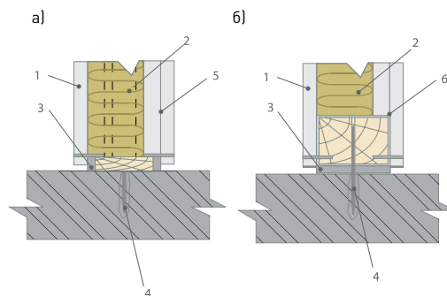
Рис. 2.3. Опираение перегородок на междуэтажное перекрытие: а — перегородка с металлическим каркасом; б — перегородка с деревянным каркасом: 1 — гипсокартонный лист; 2 — плиты ROCKWOOL АКУСТИК БАТТС®; 3 — уплотнительная лента; 4 — самонарезающий винт; 5 — горизонтальная металлическая направляющая каркаса; 6 — деревянный брусок 60x50 мм.
