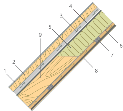
Рис. 7.3. Покрытие мансарды:
