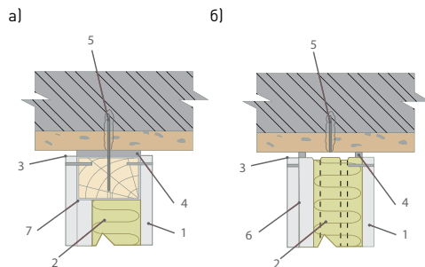
Рис. 2.2. Примыкание перегородок к верхнему перекрытию: а — с деревянным каркасом; б — с металлическим каркасом: 1 — гипсокартонный лист; 2 — плиты ROCKWOOL АКУСТИК БАТТС®; 3 — шпаклевка; 4 — уплотнительная лента; 5 — дюбель; 6 — горизонтальная металлическая направляющая каркаса; 7 — деревянный брусок 60x50 мм;
