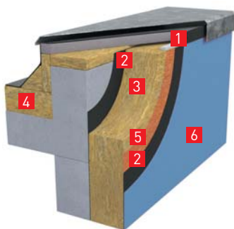
2. Узел сопряжения фасадной системы с кровлей
