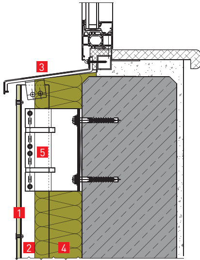
15. Нижнее примыкание фасадной системы к оконному проёму
